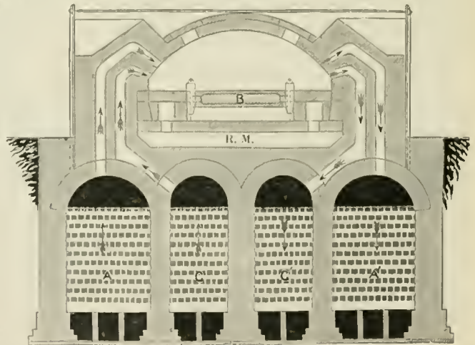
Fig. 8.—Cross Section on YY, fig. 7.
